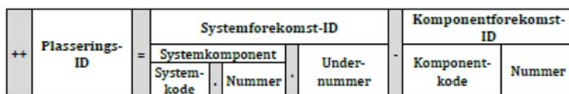
Figur 4 — Oppbygging av Minimum TFM-ID i fysisk merking
